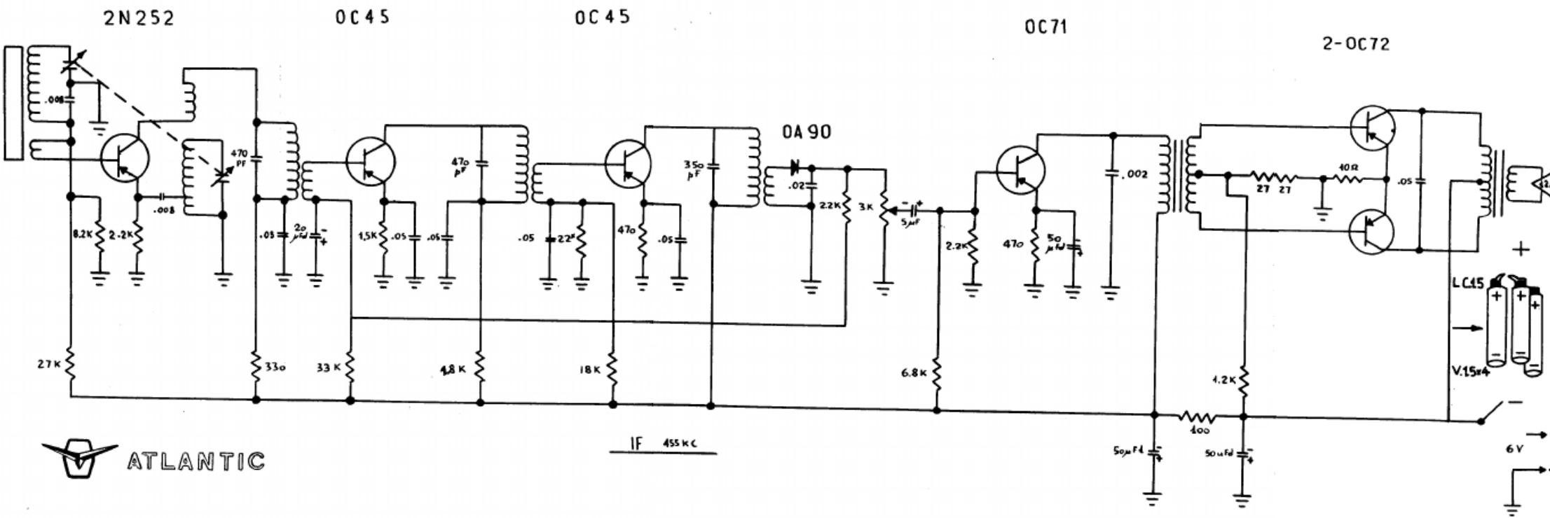
ATLANTIC ELETTRIC - Mod. T66. Apparecchio portatile a sei transistor, per la gamma delle onde medie, con antenna magnetica incorporata. Media frequenza a 455 kc/s. Resa d'uscita 100 milliwatt.
